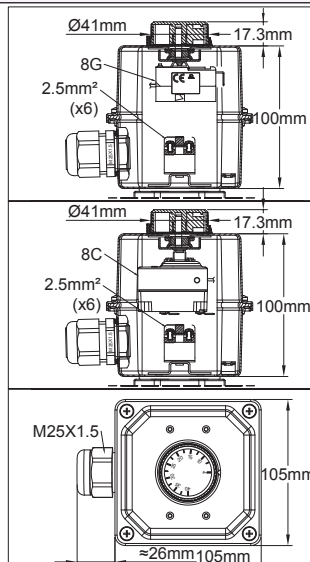
单极和3极温控器，外部 旋钮调节（可选项）
