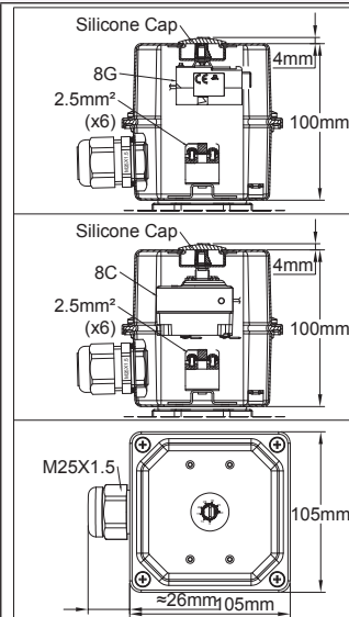
单极和3极温控器，内部 旋钮调节，在硅胶帽盖下 进入调节（标准型号）
